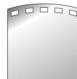
H 86 x B 80 cm Bogenhöhe 6 cm Arch rise 6 cm
